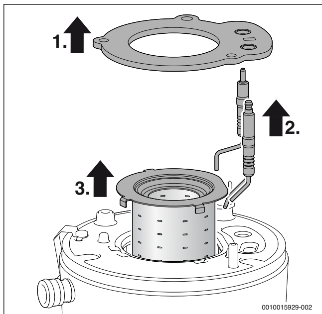
Obr. 43 Demontáž horáka
