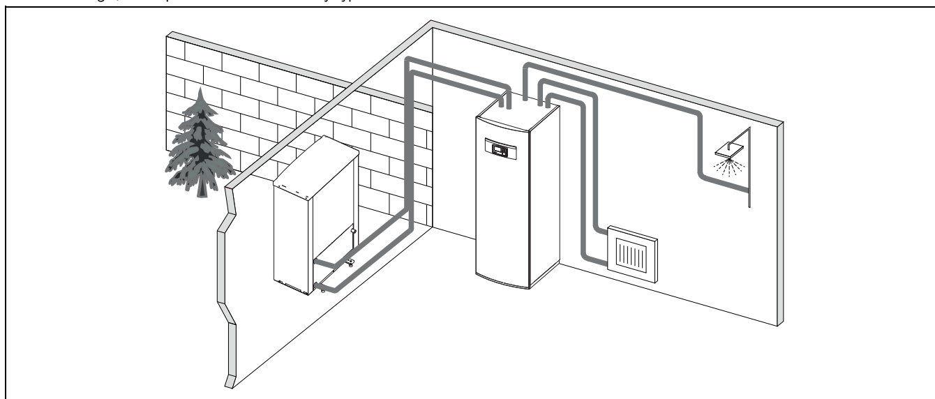
Obr. 3 Tepelné čerpadlo WPL AR, vnútorná jednotka IDU T/ IDU TS s integrovaným zásobníkom teplej vody a elektrickou vložkou pre dohrev
