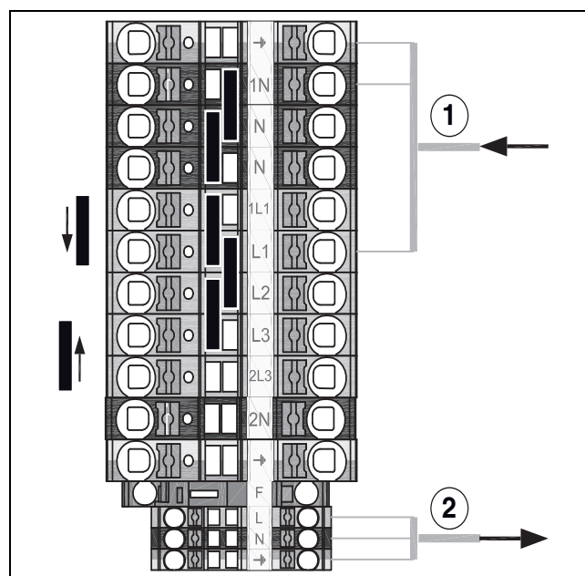
Obr. 16 1N~ vyhotovenie
