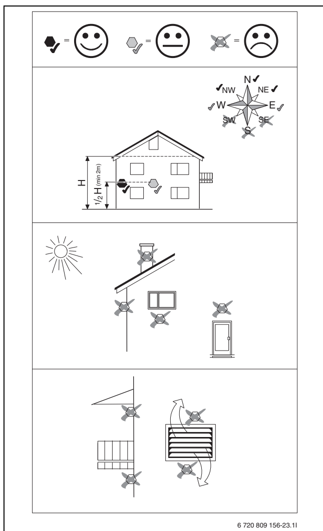
Obr. 12 Umiestnenie snímača vonkajšej teploty
