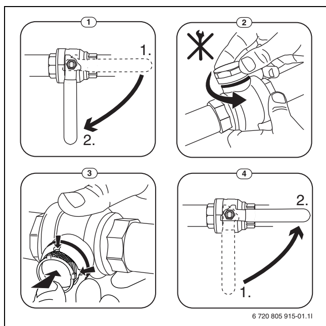
Obr. 7 Čistenie sitka
