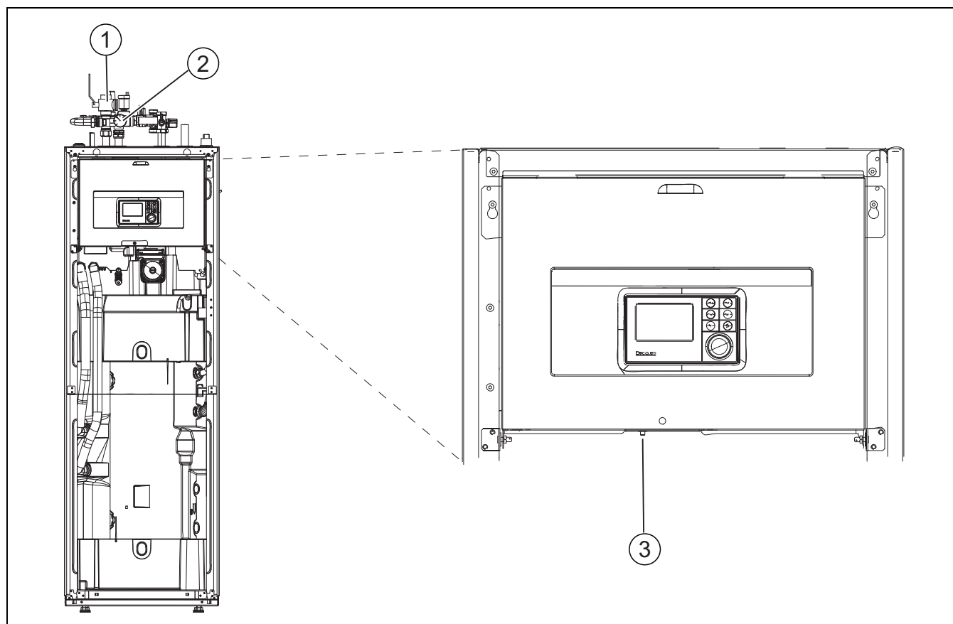
Obr. 6 Vnútoraná jednotka IDU T/ IDU TS
