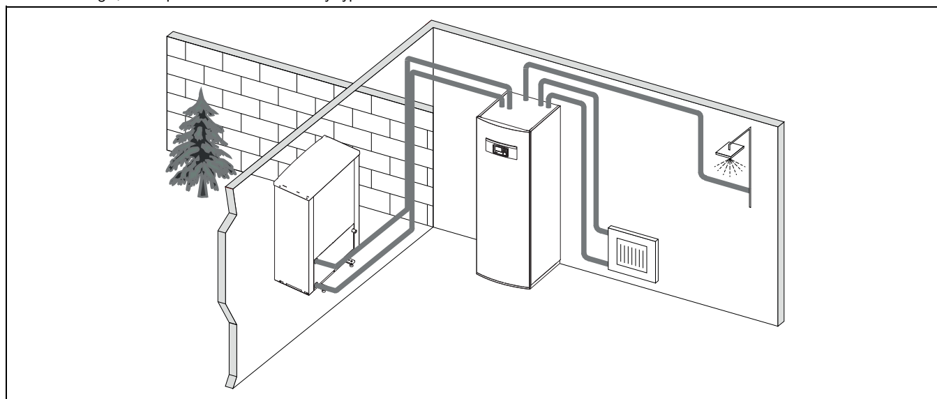
Obr. 3 Tepelné čerpadlo WPL AR, vnútna jednotka IDU T/ IDU TS s integrovaným zásobníkom teplej vody a elektrickou vložkou pre dohrev
