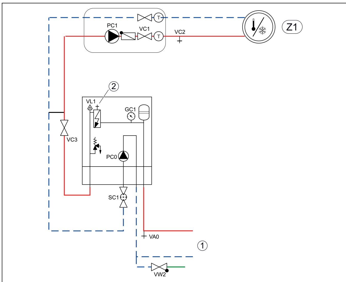
Obr. 7 Vnútroiná jednotka s integrovanou elektrickou vložkou pre dohrev
