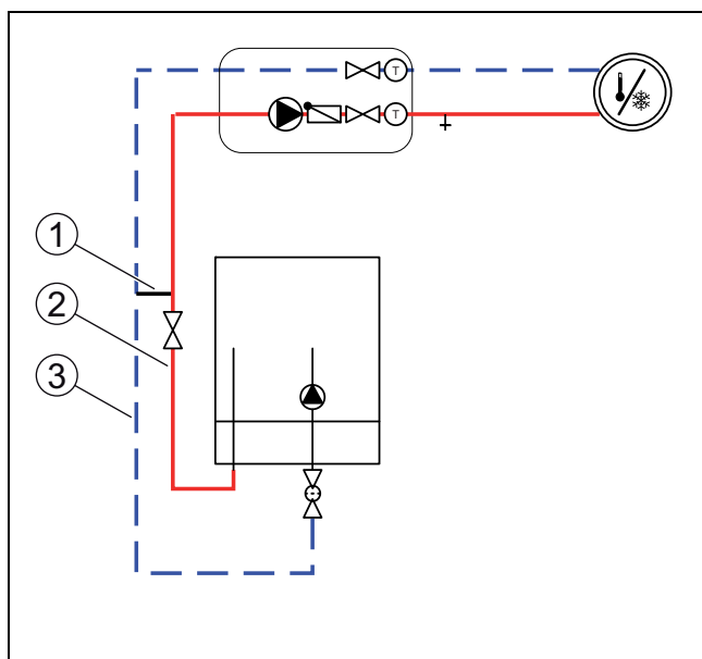
Obr. 29 Vnútrná jednotka s vykurovacím okruhom a obtokom
