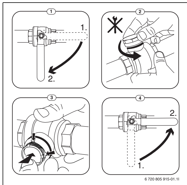
Obr. 20 Čistenie sitka
