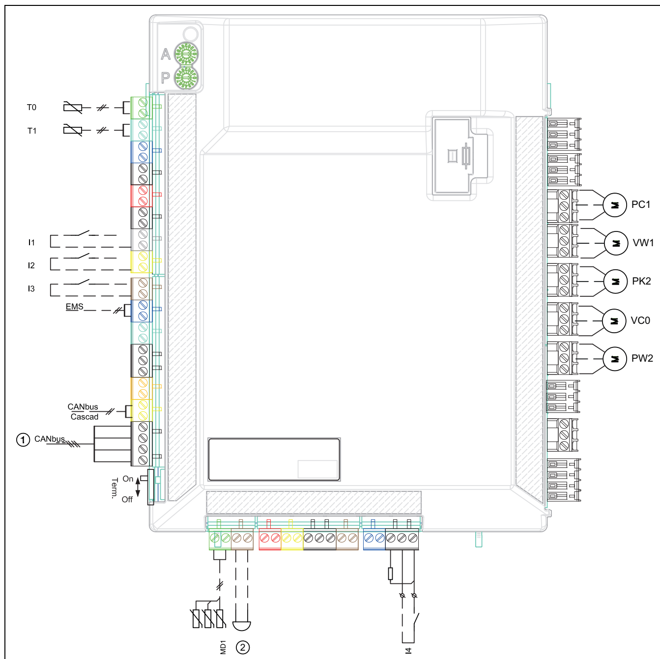
Obr. 13 Prípojky inštalračného modulu
