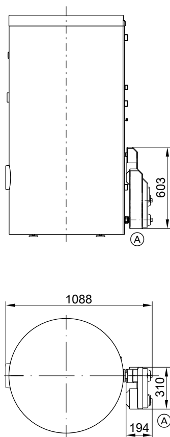
(A) Souprava solárního výměníku tepla
