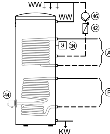
Hydraulické schéma při použití ohřivačů Vitocell 100-B, typ CVB nebo Vitocell 100-W, typ CVBC, 300 l (jako bivalentní zařízení) nebo Vitocell 100-W, typ CVAB, 300 l
