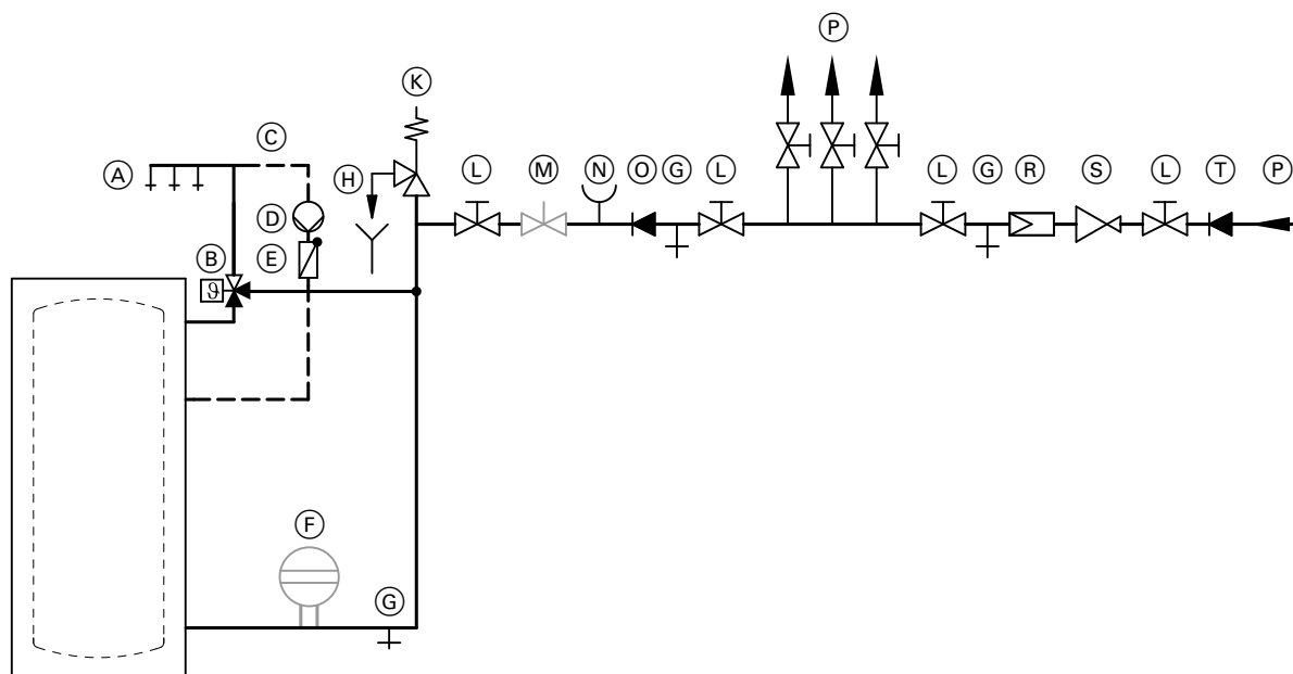
Příklad s ohřívačem Vitocell 100-V/100-W, typ CVWA/CVWB
