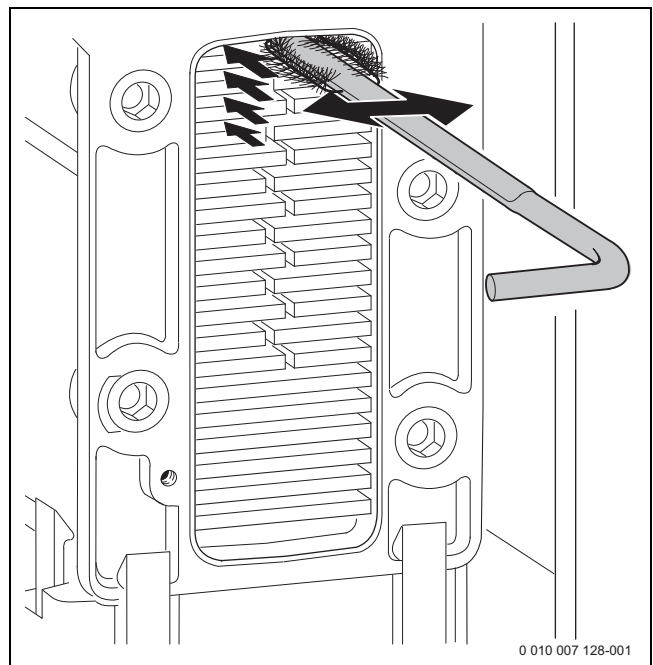
Obr. 52 Čistenie tepelného bloku kefou
