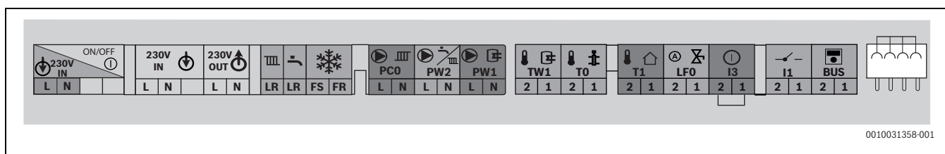
Obr. 35 Svorkovnica pre externé príslušenstvo
