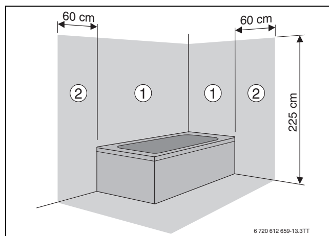
Obr. 20 Ochranné zóny
