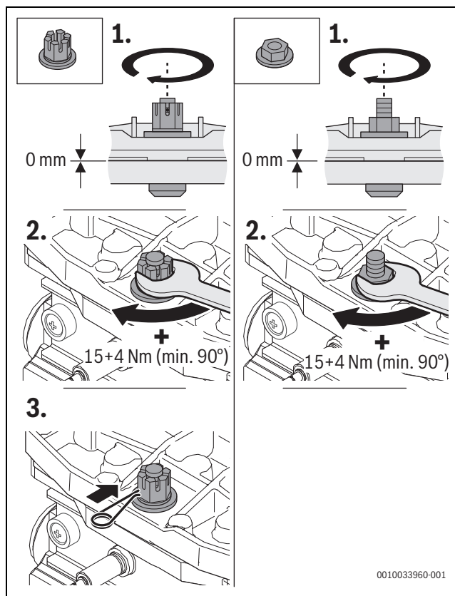
Obr. 47 Pritiahnutie matice na kryte horáka
