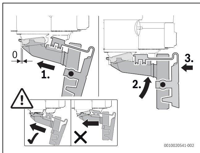
Obr. 58 Montáž sifónu na kondenzát
