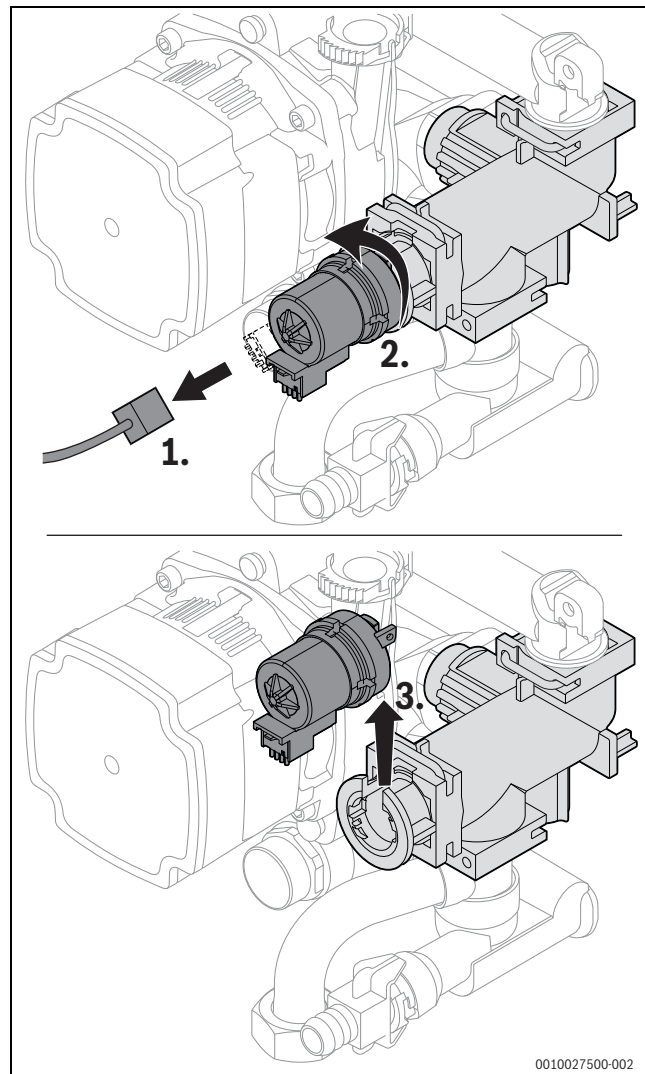
Obr. 62 Demontáž motora na 3-cestnom ventile (verzia bez skrutiek)
