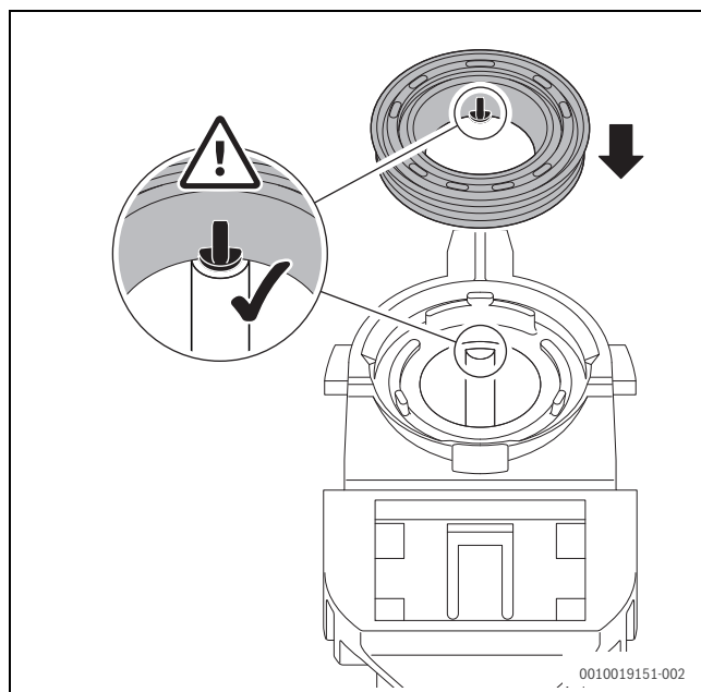
Obr. 56 Vyrovnanie nového tesnenia na sifóne na kondenzát
