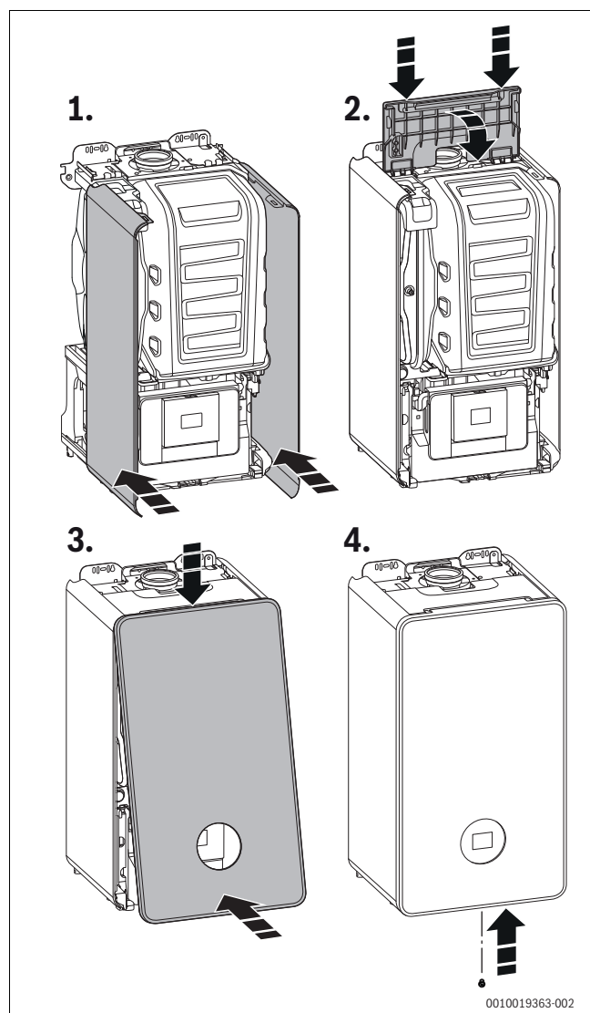
Obr. 36 Montáž plášt'a
