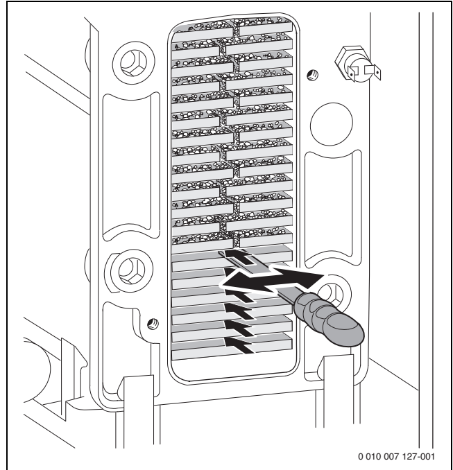
Obr. 51 Čistiaci nôž
