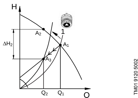
Obr. 8 Čerpadlo regulované na proporcionální tlak
