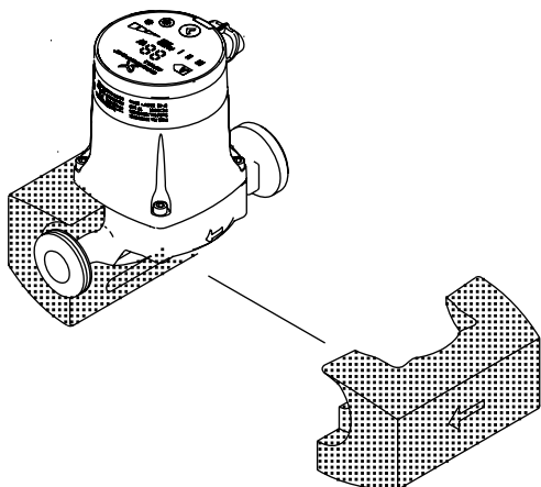
Obr. 18 Tepelně-izolační kryty
