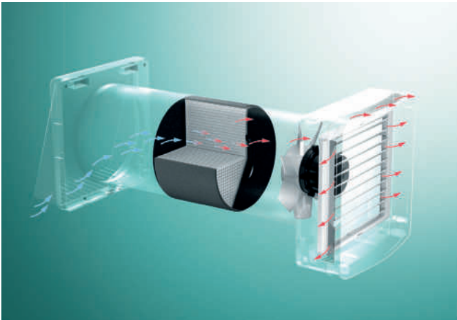
Rekuperácia tepla prostredníctvom keramického výmenníka tepla
