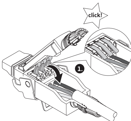
Fig. 27: Jousilukkojen sulkeminen
