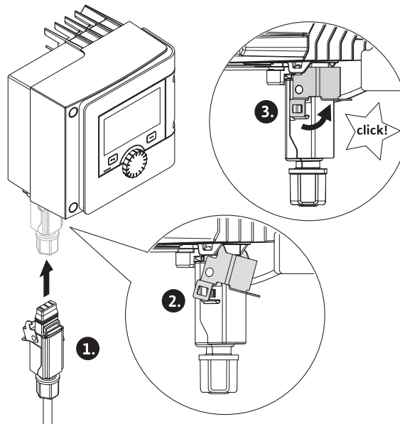
Fig. 29: Wilo-Connector montieren
