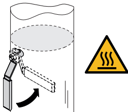
Fig. 14: Κλείσιμο βαλβίδων απομόνωσης
