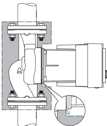
Fig. 20: Isoler, la kondensatavløp være fritt
