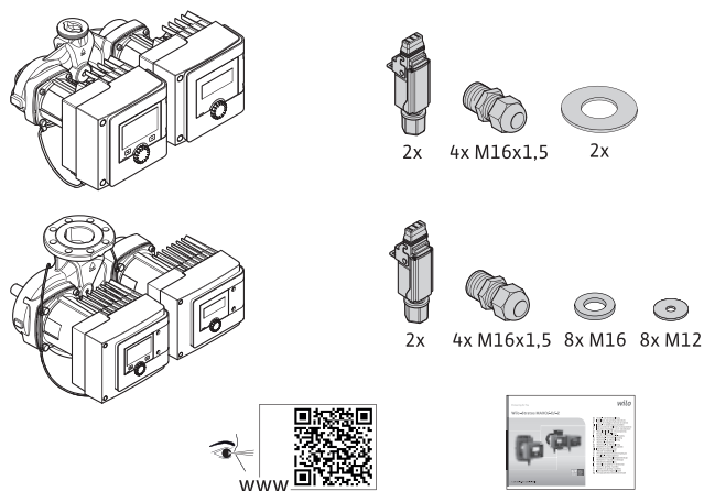
Fig. 7: Leveransomfattning tvillingpumpar
