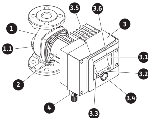
Fig. 1: Vakiopumpun yleiskatsaus
