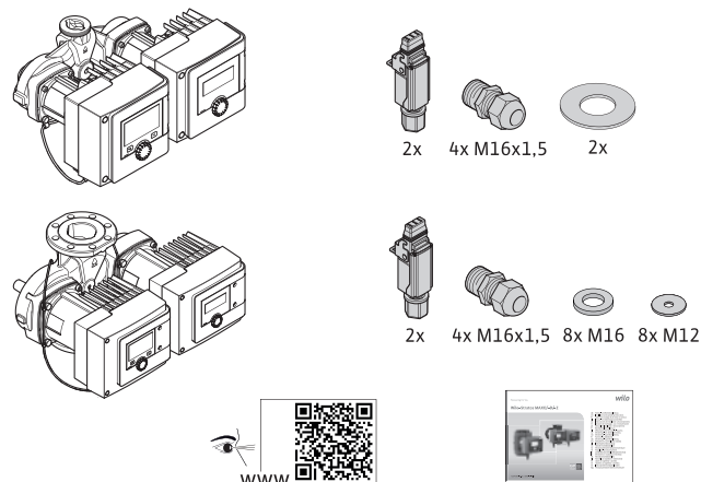
Fig. 7: Leveringsomfang dobbelpumper
