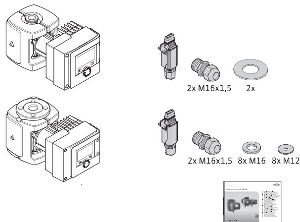
Fig. 6: Leveringsomfang enkeltpumper
