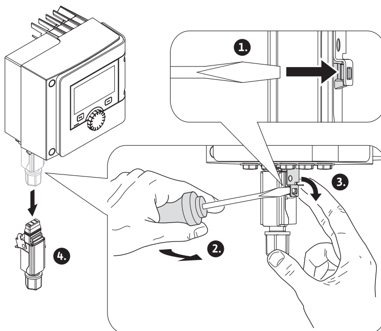
Fig. 30: Afmontering af Wilo-Connector
