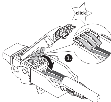
Fig. 27: Затваряне на пружинната клем
