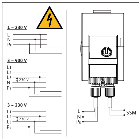
Obr. 14: Možnosti pripojenia
