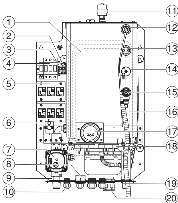
Obr. 2 Funkčné prvky kotla Tronic Heat 3000/ Tronic Heat 3500 15-24 kW
