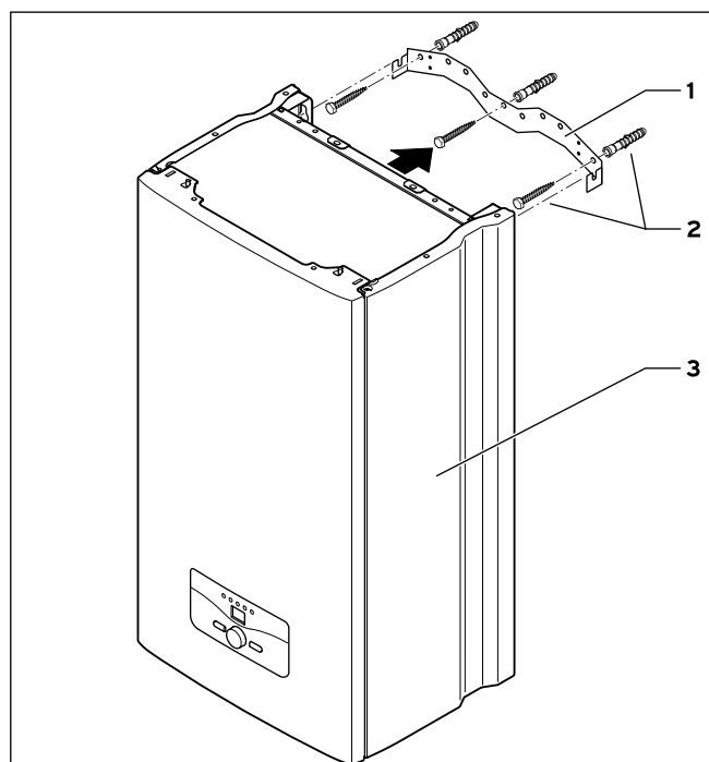
4.5 Zavesenie výrobku
