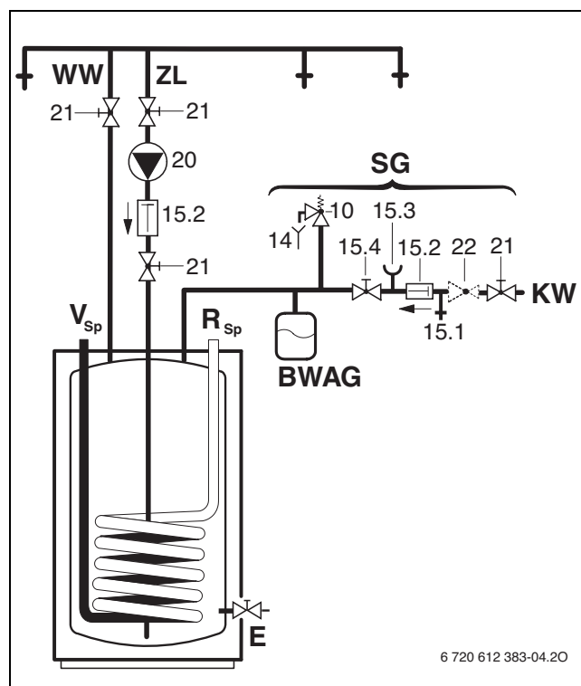
Obr. 4 Schéma pripojenia pitnej vody
