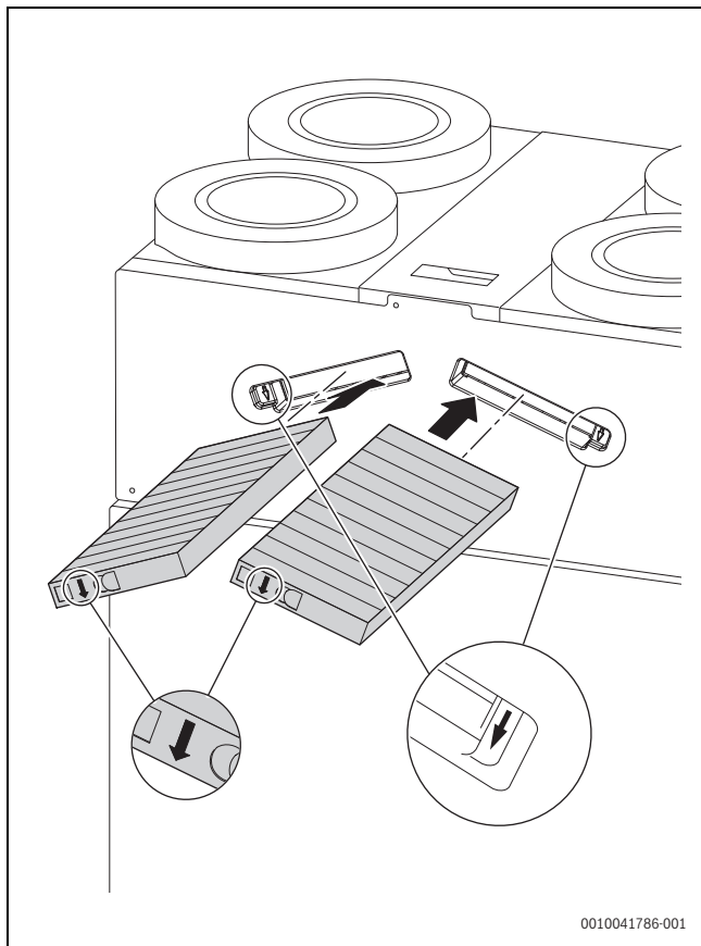
Obr. 8 Vloženie filtra
