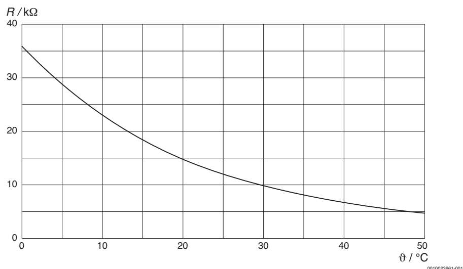
Obr. 66 Charakteristika TV1 (12K)
