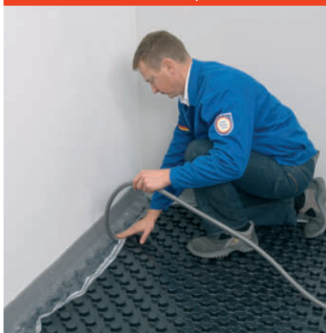
Obr. 8: Pokládka kruhového PE-profilu
