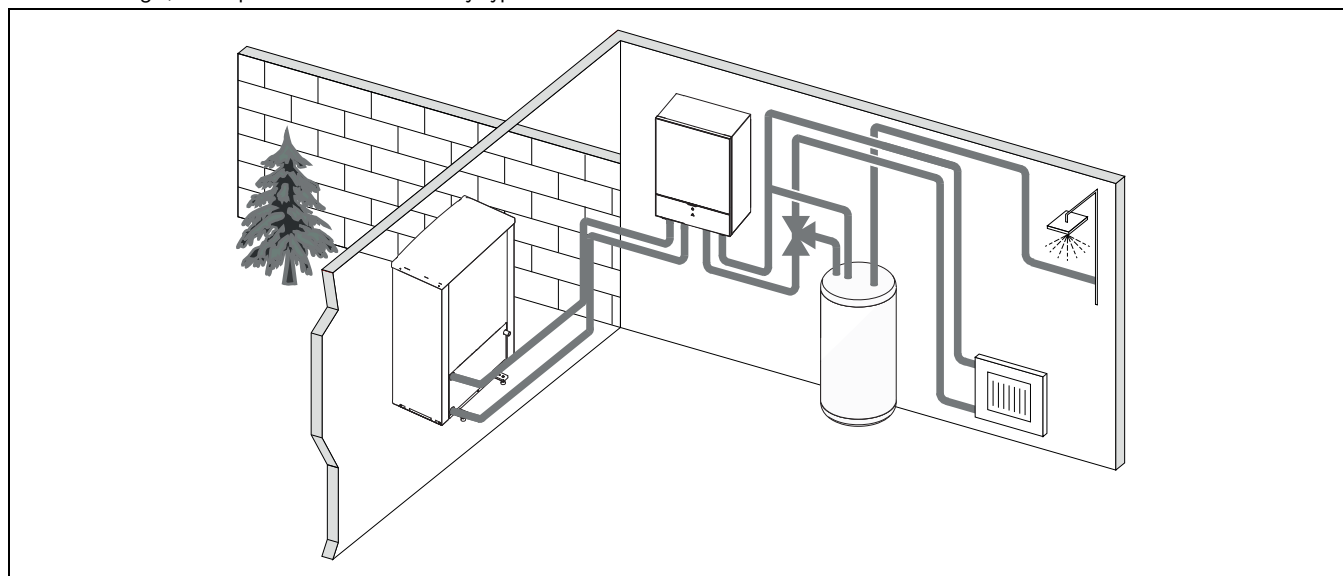
Obr. 3 Tepelné čerpadlo WLW196i AR, vnútorná jednotka IDU-..iE s elektrickou vložkou pre dohrev a externým zásobníkom teplej vody
