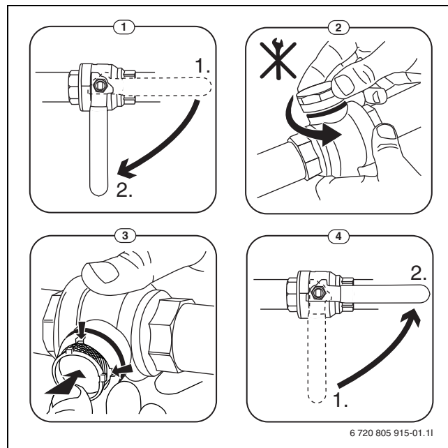
Obr. 8 Čistenie sitka
