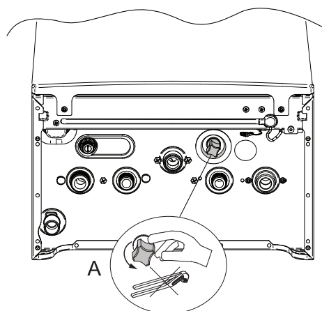
Obr.44 Plnenie systému (inštalácie)
