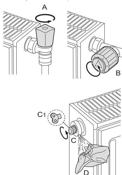
Fig.36 Purjarea instalației
