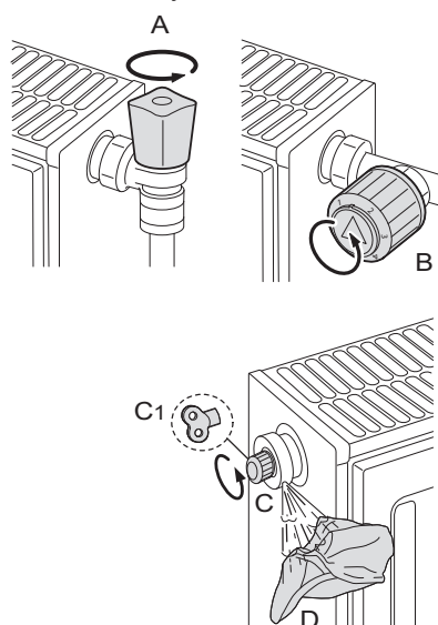
Obr.45 Čistenie systému
