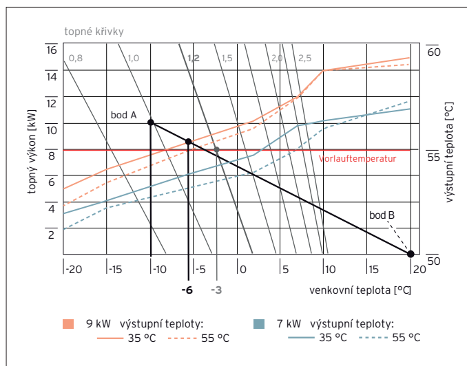
Výpočet bivalentního bodu pro tepelné čerpadlo
