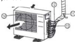
Venkovní jednotka
