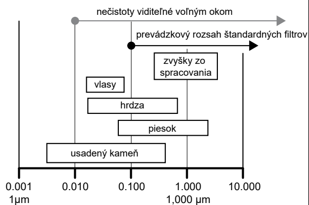
prevádzkový rozsah odľučovača mikro nečistôt / špiny
