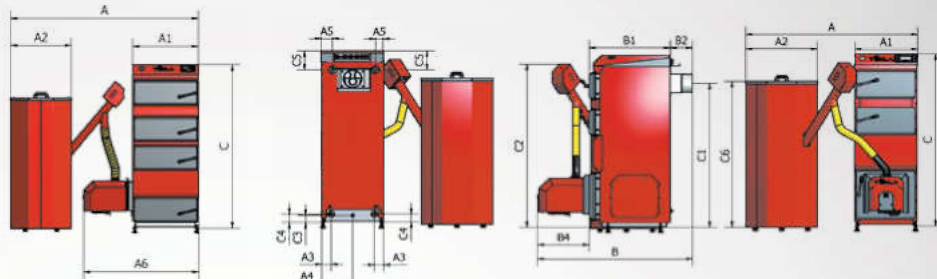
ROZMERY DRACO D BIO 50
