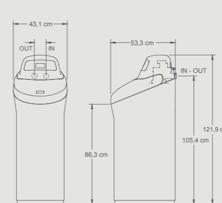
NSC42 ECOMULTI
