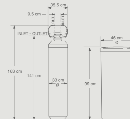
NST70 ECOMULTI
