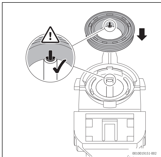
Obr. 60 Vyrovnanie nového tesnenia na sifóne na kondenzát
