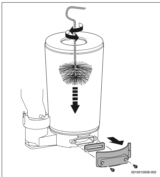
Obr. 46 Čistenie tepelného bloku
