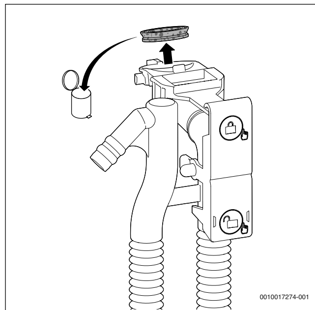
Obr. 51 Vymeňte tesnenie v hornej časti sifónu na kondenzát
