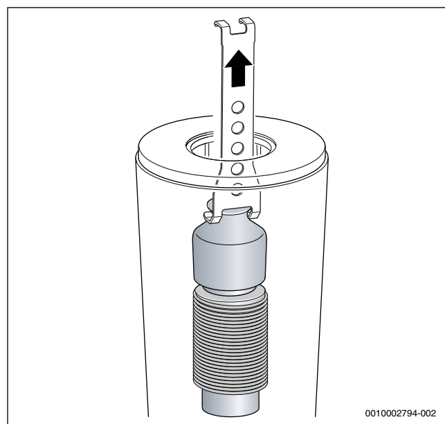
Obr. 44 Demontáž horného výtláčného telesa
