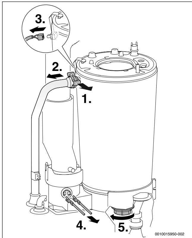
Obr. 63 Uvoľnenie potrubia výstupu a stiahnutie kábla
