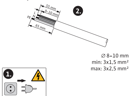
Fig. 24: Προετοιμασία σύνδεσης
