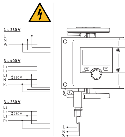
Fig. 23: Tilkoblingsmuligheter
