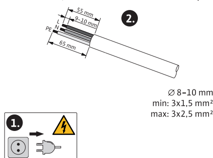
Fig. 21: Liitännän valmistelu
