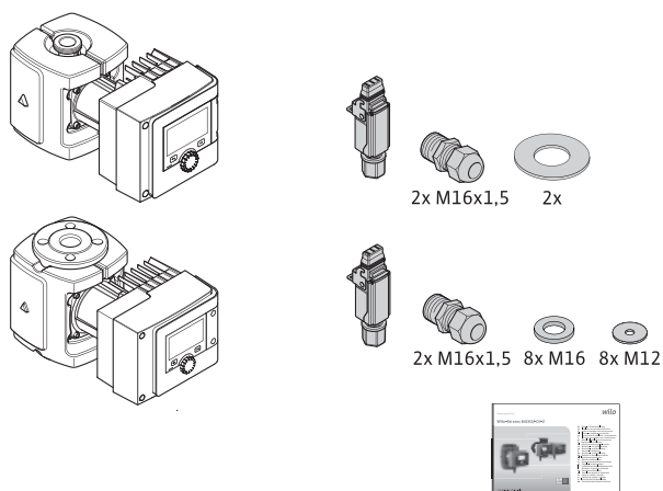
Fig. 6: Περιεχόμενο παράδοσης μεμονωμένων αντλιών
