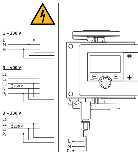
Fig. 23: Δυνατότητες σύνδεσης
