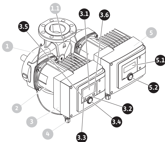
Fig. 36: Käyttölaitteet (kaksoispumppu)
