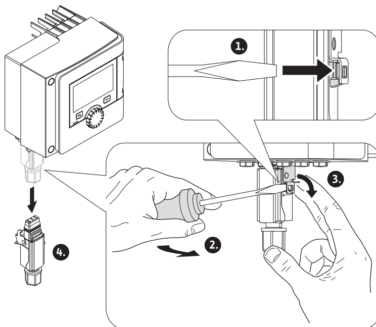
Fig. 30: Demontáž Wilo-Connectoru
