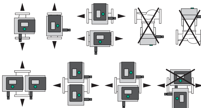
Fig. 3: Tilladte installationspositioner
