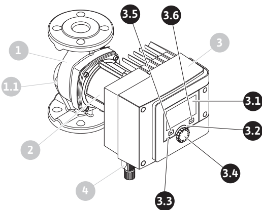
Fig. 35: Bedieningselementen (enkelpomp)
