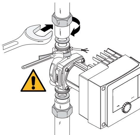
Fig. 12: Συναρμολόγηση αντλίας
