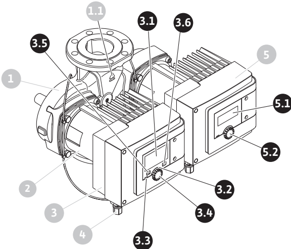
Fig. 36: Bedieningselementen (dubbelpomp)
