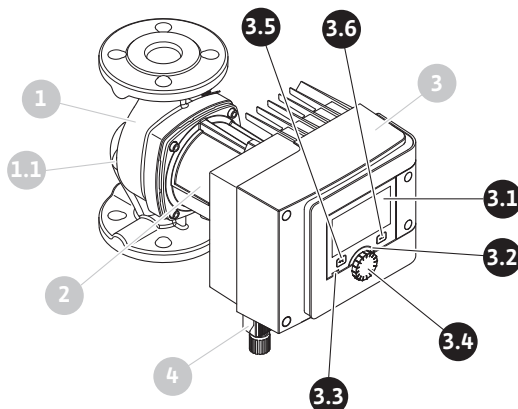
Fig. 35: Juhtelementid (üksikpump)
