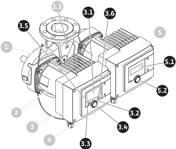
Fig. 36: Bedienelemente (Doppelpumpe)
