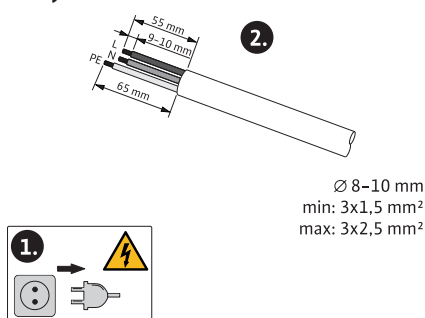
Fig. 24: Priprava priključka
