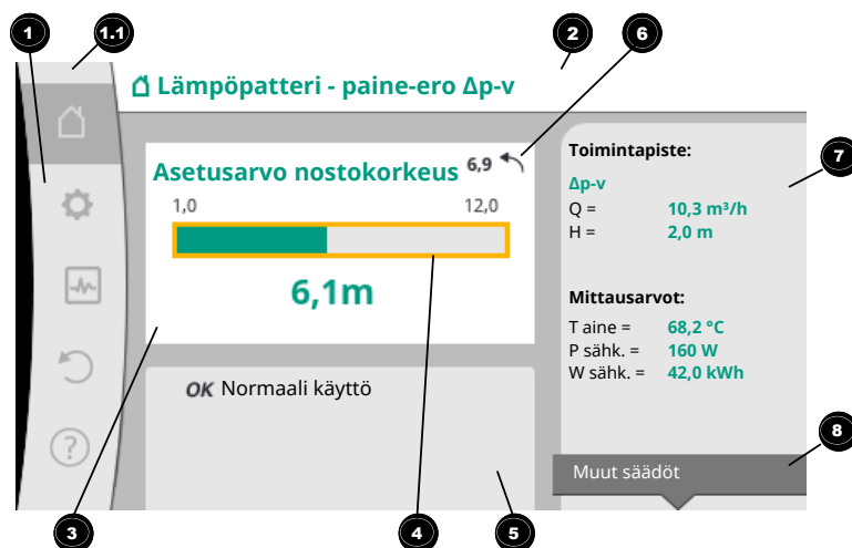
Fig. 38: Aloituspäyttö
