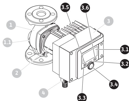
Fig. 35: Manöverelement (enkelpump)
