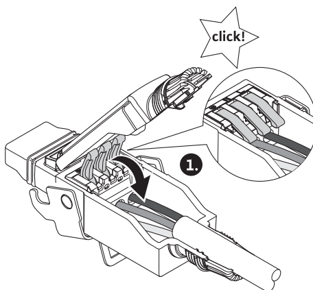
Fig. 27: Atsperspailes aizvēršana
