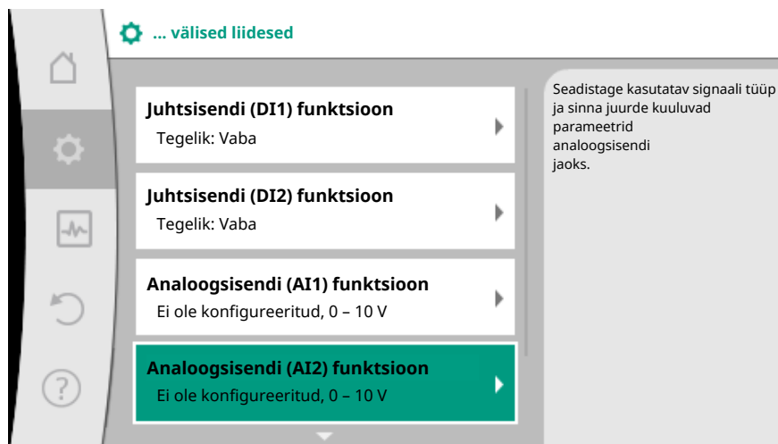
Fig. 62: Analoogsisendi funktsioon
