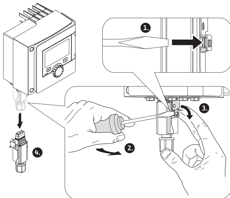
Fig. 90: Wilo-Connector-liittimen irrotus
