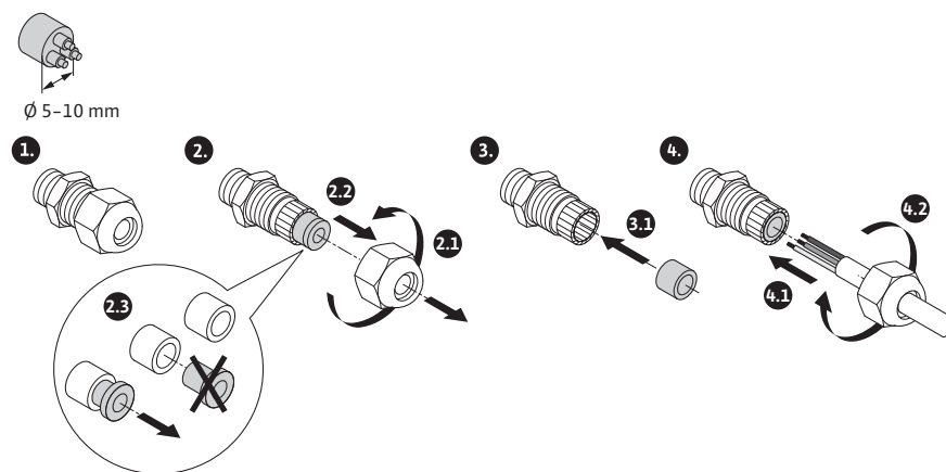
Fig. 22: Kabelschroefverbinding \varnothing 5 - 10 mm
