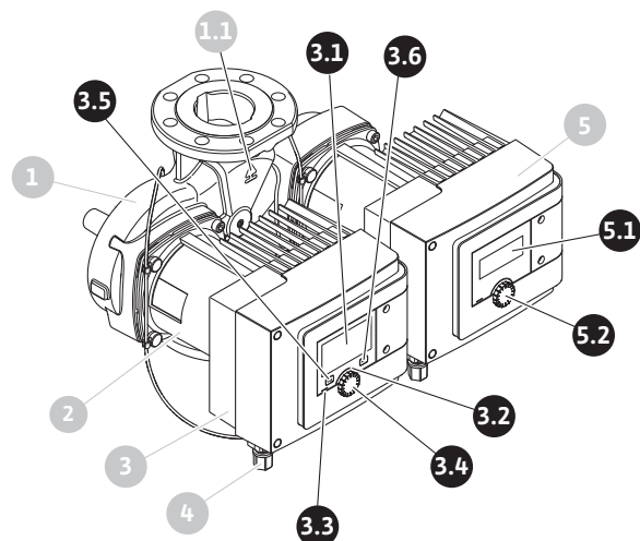
Fig. 36: Manöverelement (tvillingpump)
