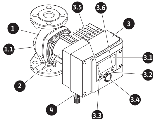
Fig. 1: Overzicht enkelpomp
