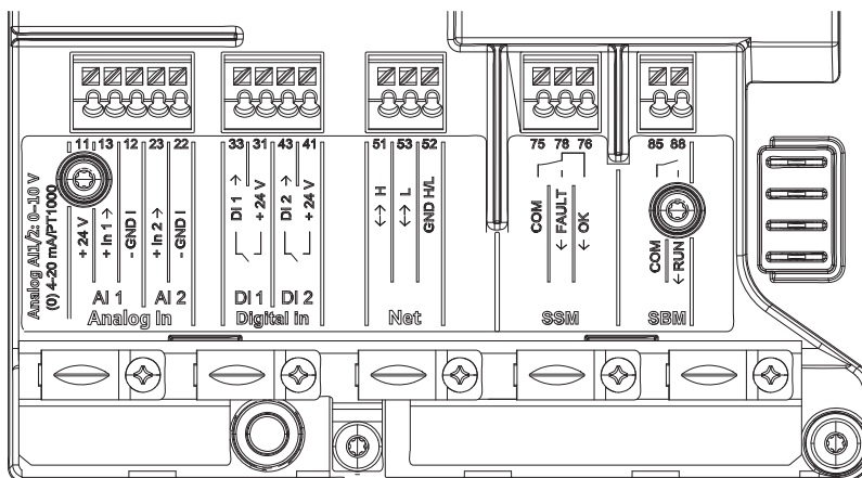
Fig. 32: Kommunikációs interfészek
