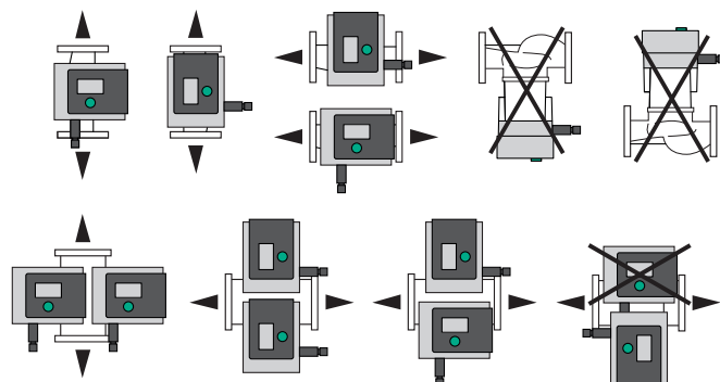
Fig. 3: Zulässige Einbaulagen
