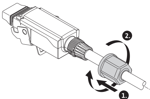
Fig. 28: Zatvorenie zástrčky
