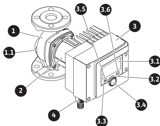
Fig. 1: Oversikt enkeltpumpe
