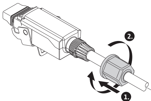
Fig. 28: Spraudņa aizvēršana
