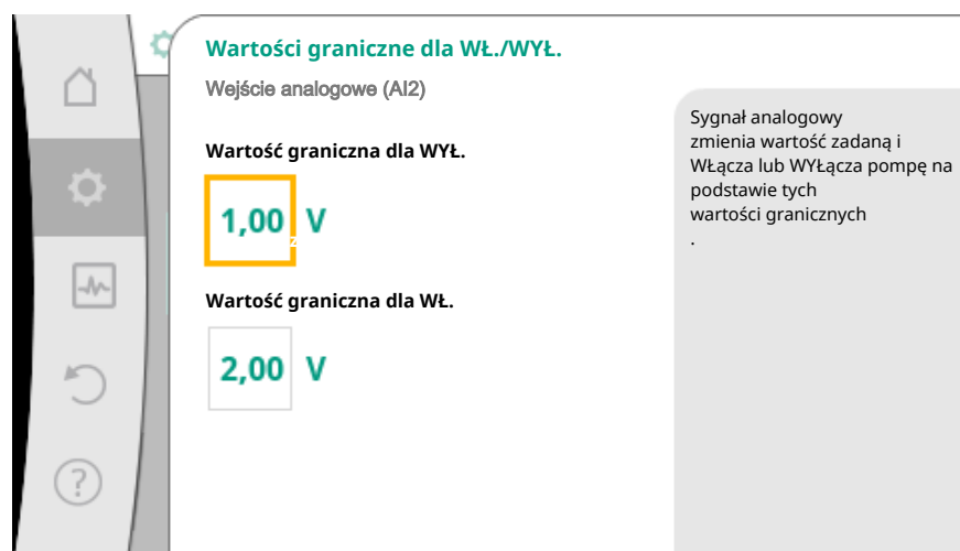
Fig. 74: Wartości graniczne sterowania WŁ./WYŁ. za pomocą sygnałów analogowych Rampa przenoszenia jest teraz zdefiniowana dla transmisji wartości sygnałów analogowych do wartości zadanych. W tym celu określa się minimalne i maksymalne punkty wsparcia charakterystyki pompy oraz związane z nimi wartości zadane (przypisanie sygnału/wartości MIN i przypisanie sygnału/wartości MAX).
