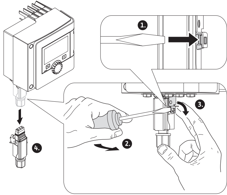
Fig. 30: Wilo-Connector'ü sökme
