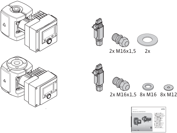
Fig. 6: Leveransomfattning enkelpumpar
