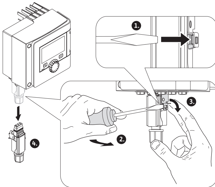
Fig. 90: Wilo-Connector demontieren
