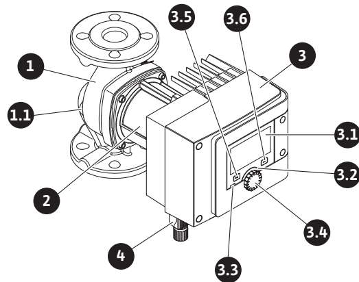
Fig. 1: Üksikpumba ülevaade
