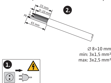
Fig. 21: Liitännän valmistelu
