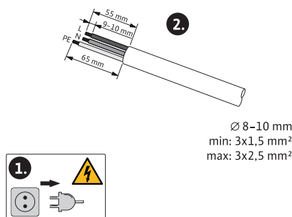
Fig. 24: Preparazione dell'allacciamento
