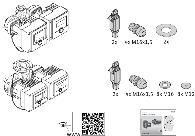
Fig. 7: Leveringsomfang dobbelpumper
