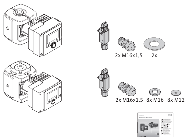
Fig. 6: Leveringsomvang enkelpompen
