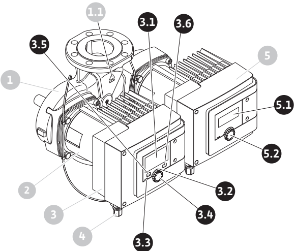
Fig. 36: Betjeningselementer (dobbeltpumpe)
