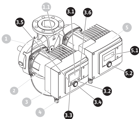
Fig. 36: Käyttölaitteet (kaksoispumppu)
