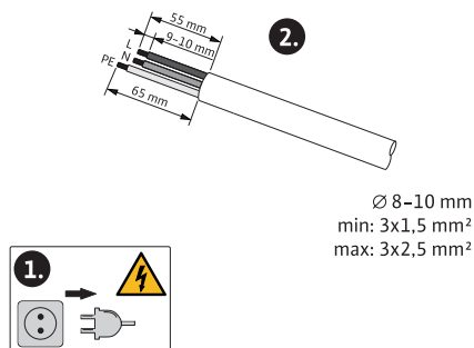
Fig. 24: Preparazione dell'allacciamento
