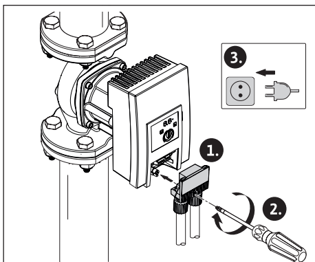
Obr. 21: Montáž zástrčky
