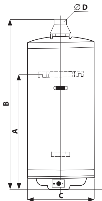
Obr. 1: Základné rozmery zásobníkov vody
