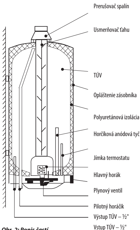
Obr. 2: Popis častí zásobníkov vody
