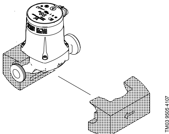
Obr. 18 Tepelně-izolační kryty
